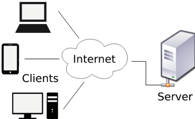
Рис. 1. Архітектура “клієнт-сервер”.
