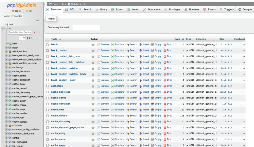
Рис. 2. Інтерфейс PHPMyAdmin
