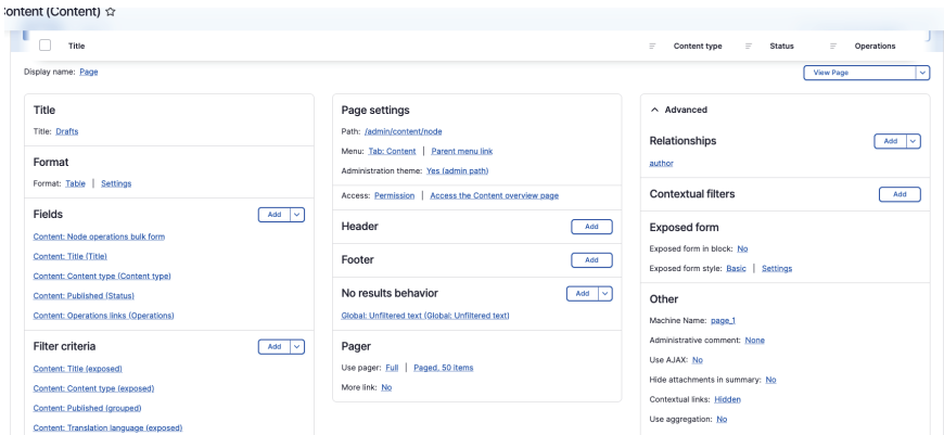
Рис. 4. Інтерфейс Views
